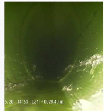
Kanalsanierung - Eiprofil SWK
